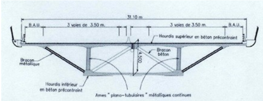
(Coupe transversale du tablier)
