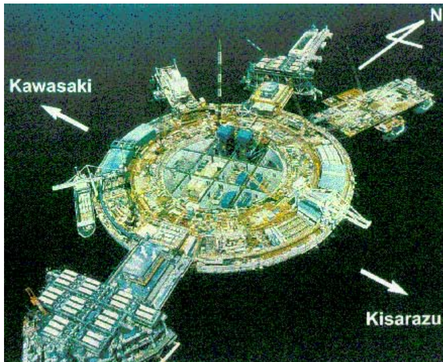
île sur le tracé du tunnel routier à travers la baie de Tokyo
