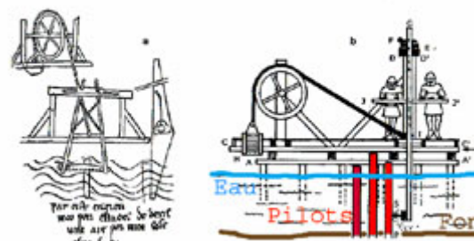
Appareil pour couper les pilots sous l'eau dans les carnets de dessins de Villars de Honnecourt (XIII e siècle)
