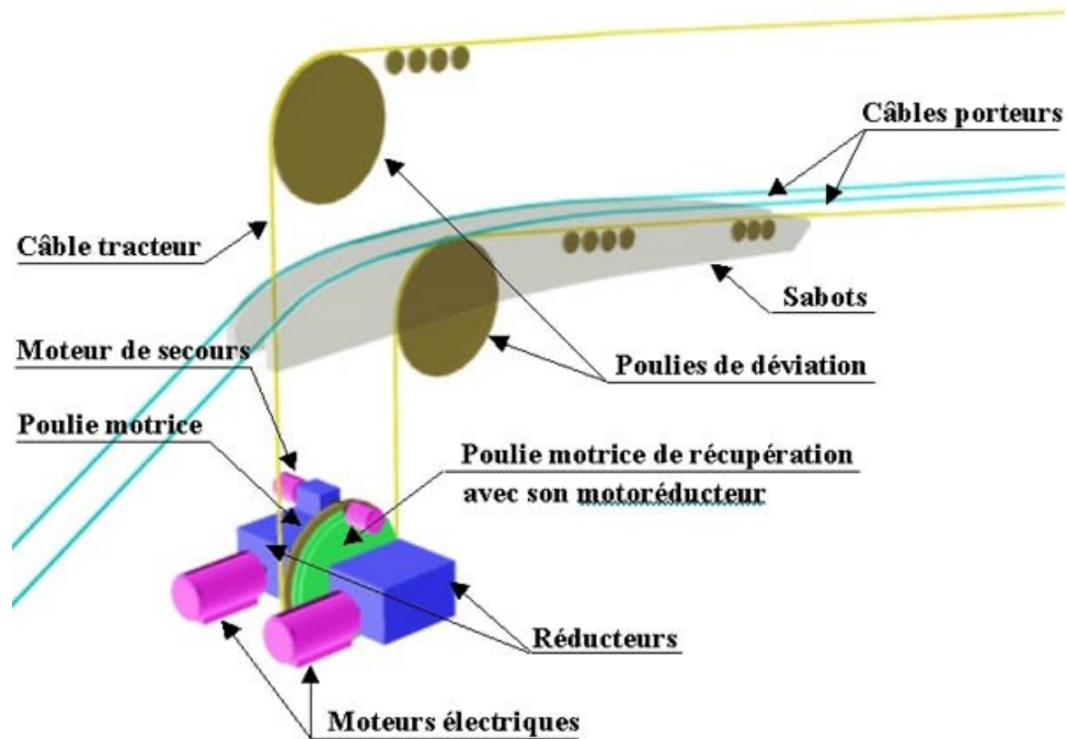
Ensemble motorisation-freinage de la gare des Arcs (Gare motrice)
