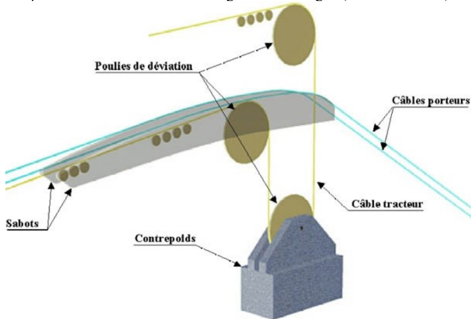
Ensemble contrepoids des câbles tracteurs de la gare de La Plagne (Gare de tension)
