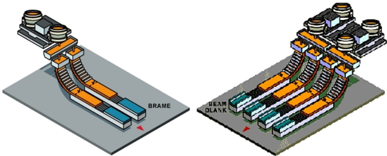
Coulée continue - moulage d'une brame (Arcelor)
