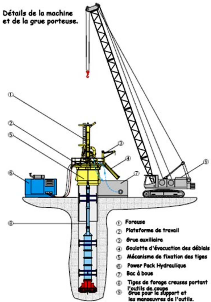
Schéma de l'ensemble de la machine (Doc Wirth – Droits réservés)
